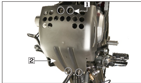
(1) Pernos (2) Placa de protección
