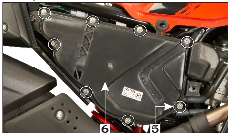
(5) Tornillos tapa filtro de aire
