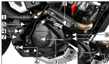
(1) Pedal de arranque (2) Cable de embrague (3) Tapa del cárter derecho (4) Tuerca del brazo oscilante (5) Perno soporte posapiés del conductor (6) Perno de la cubierta (7) Conjunto del soporte del reposapiés (8) Mangueras del enfriador de aceite (9) Pernos
