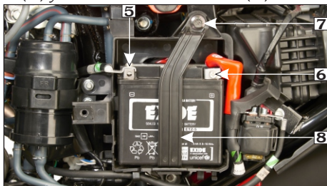
(5) Terminal (-)ve (6) Terminal (+)ve (7) Perno abrazadera (8) Abrazadera
