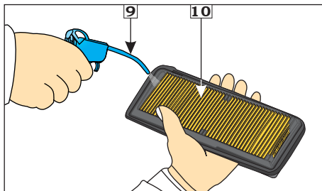
(9) Boquilla de aire
